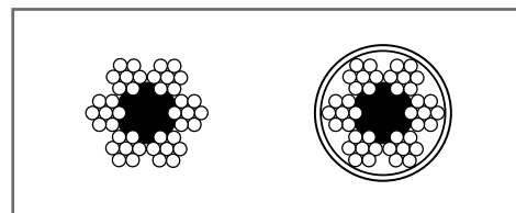
CABLES DE ACERO ACABADO GALVANIZADO - ALMA DE CAÑAMO
